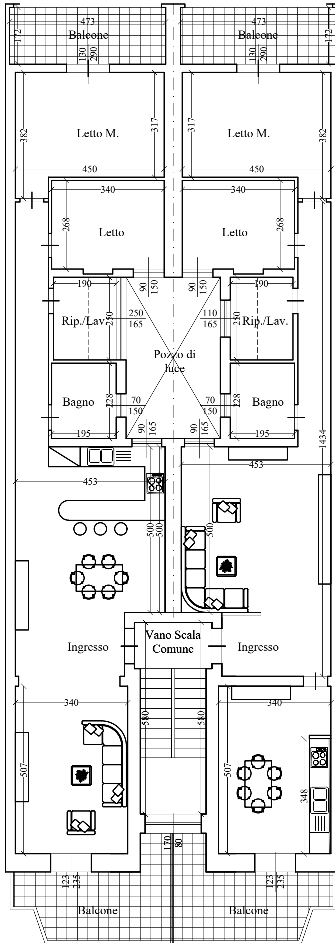
Pianta Piano Primo PROGETTO
